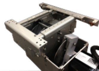
CS3000 Motor End
